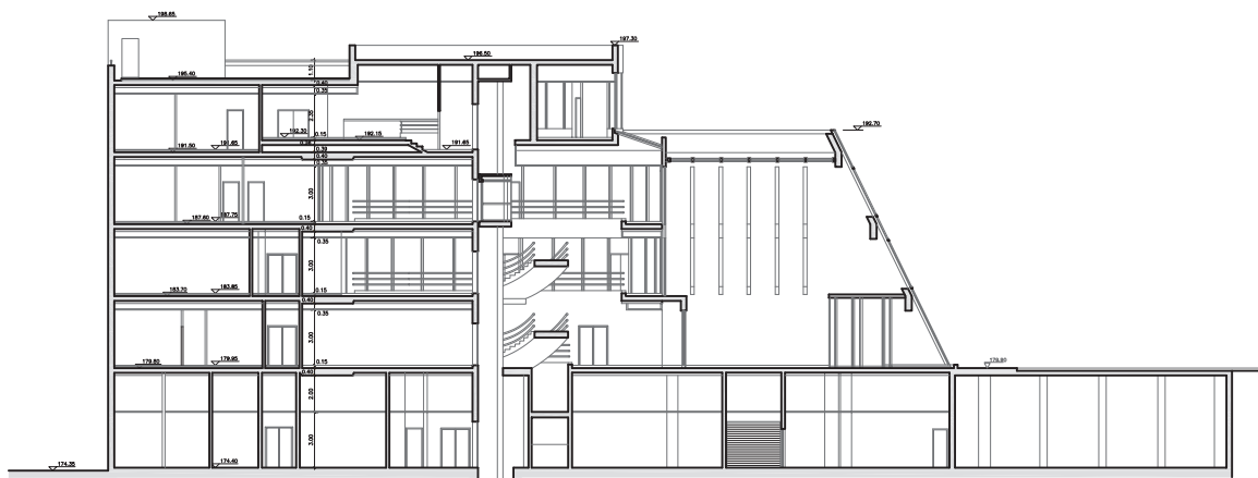
CORTE D-D
