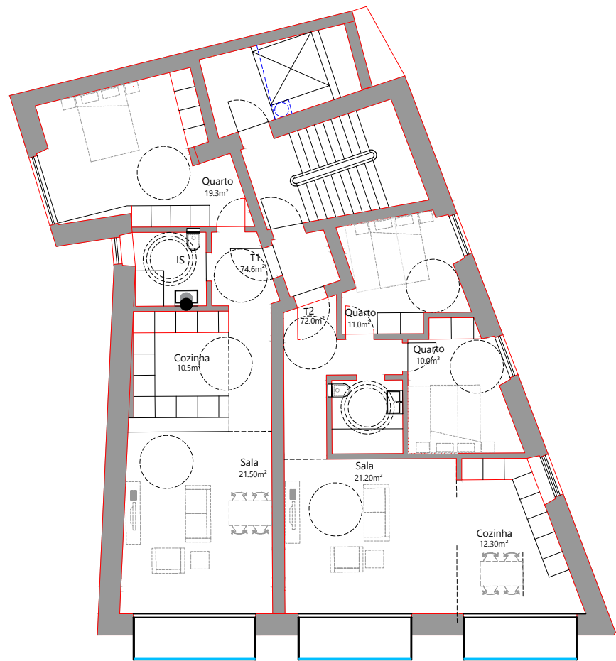
Piso 2
