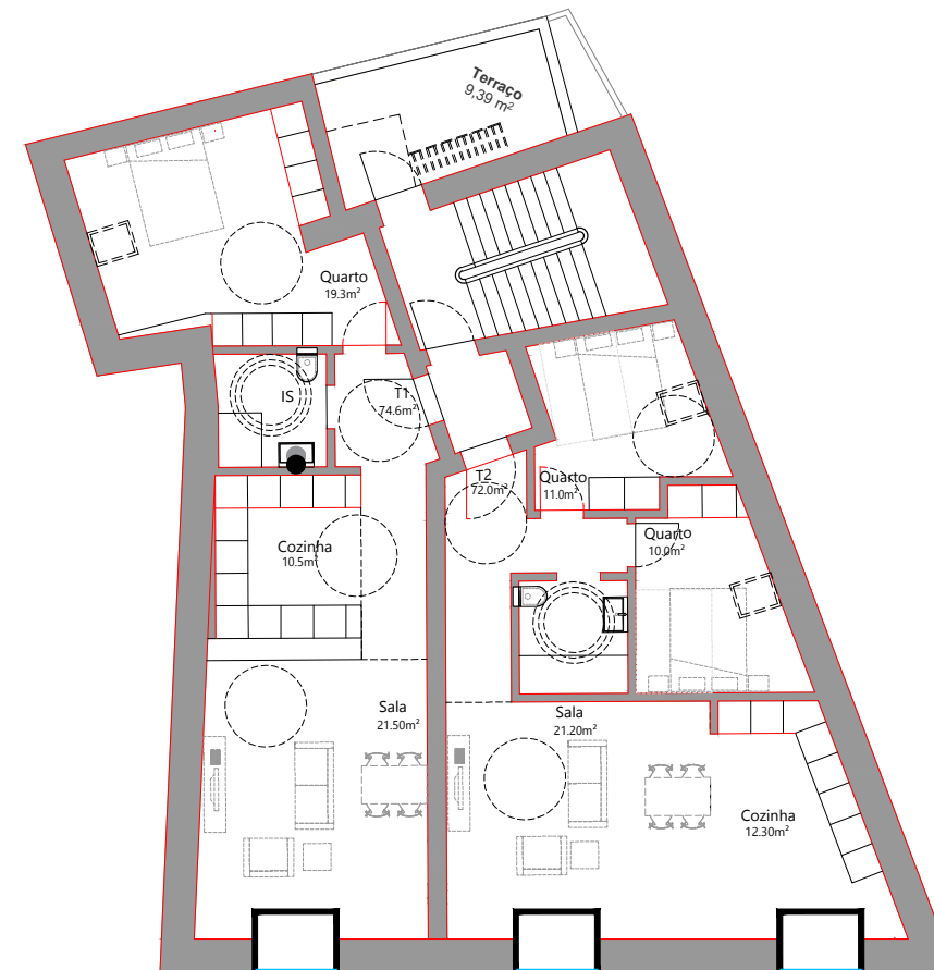
Sótão
