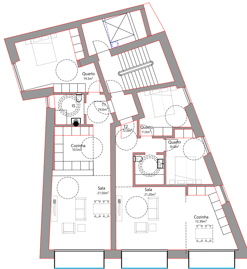
Piso 3
